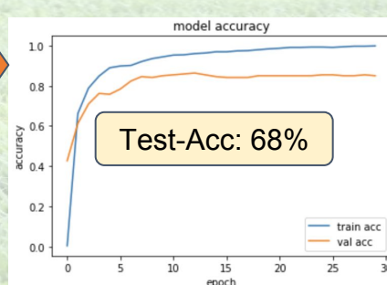
VGG16 mit Tuning
