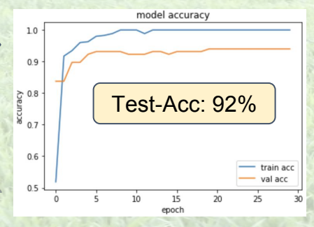
VGG16 ohne Tuning
