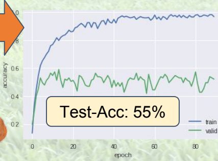
gleiches CNN mit 400 x 400 Pixel
