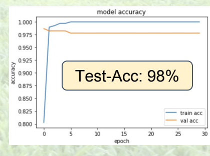
Xception
