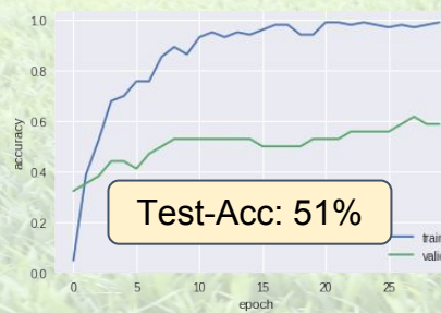
4 Layer CNN analog oben
