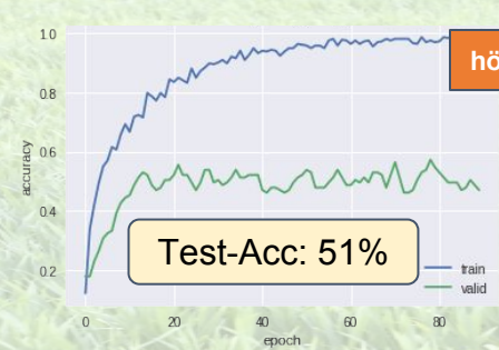
4 Layer CNN Image Augmentation 224x224
