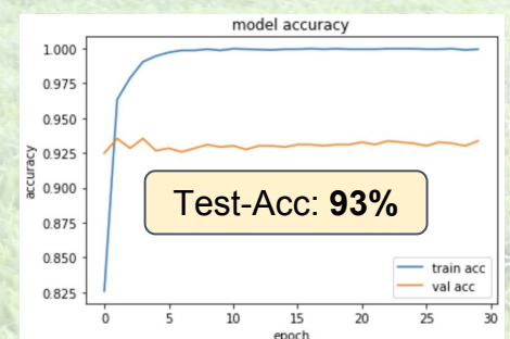
Xception
